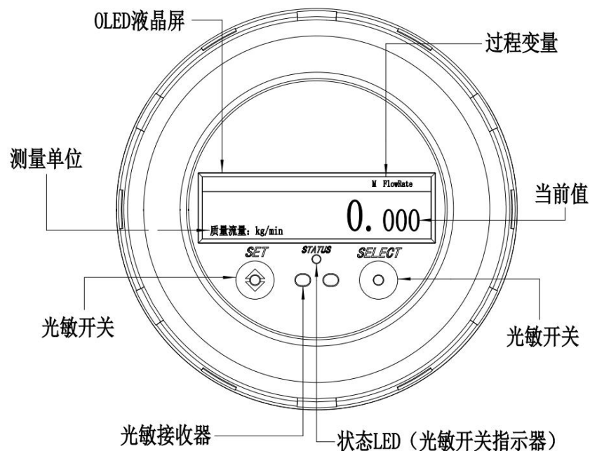
图 5-1 操作面板整体示意图
