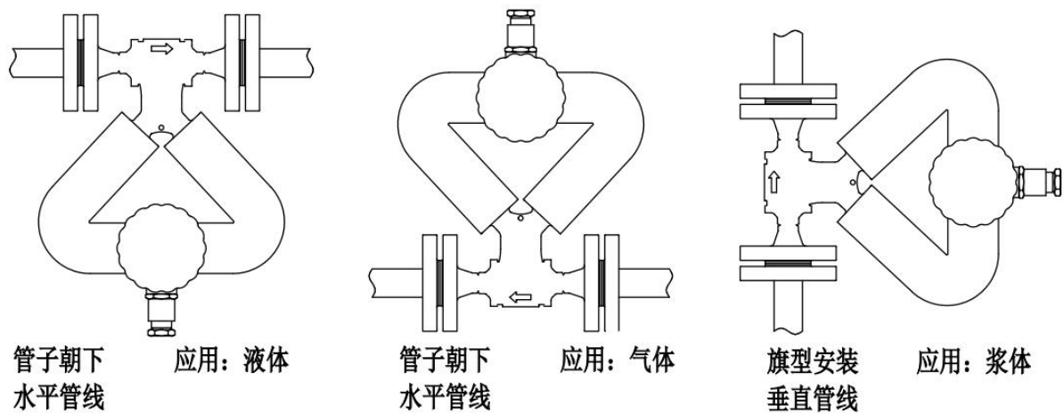
图 3-1 质量流量计管道安装示意图
