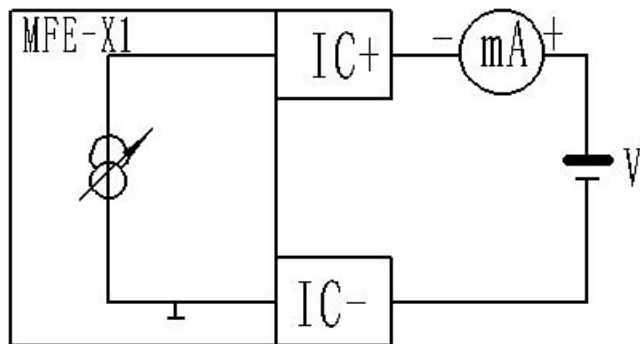
无源 4~20mA 电流输出
