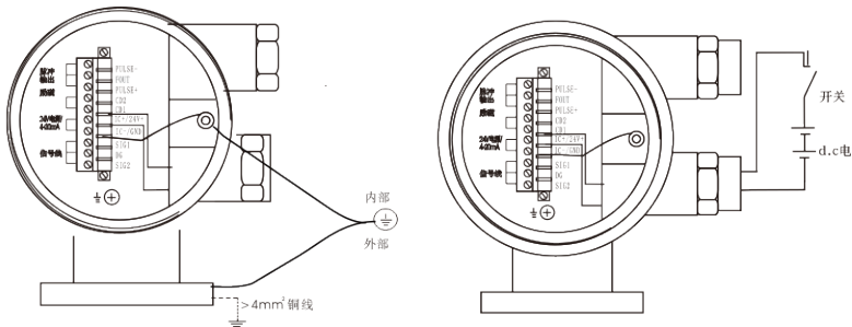
直流供电电源连接图 (DC24V)
