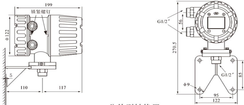
分体型转换器
