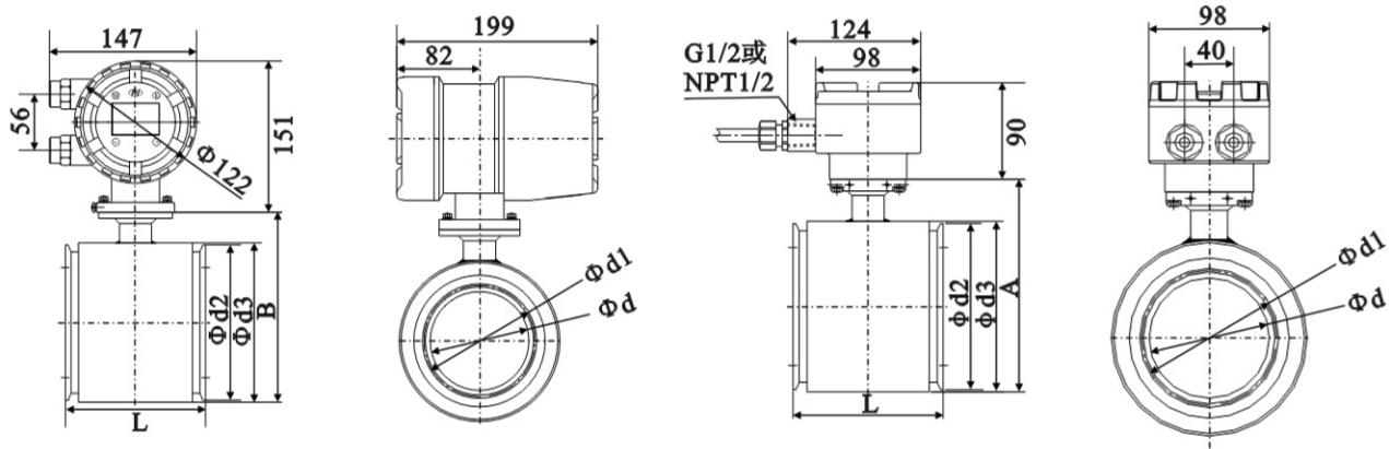
4. 2. 3. 卫生型尺寸
