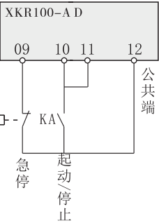
两线控制
