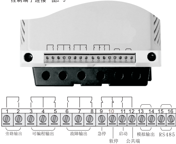
控制电路端子说明
