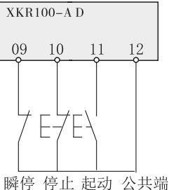
三线控制
