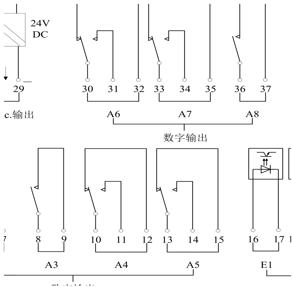
图5a 电液执行机构—对外接线端子图
