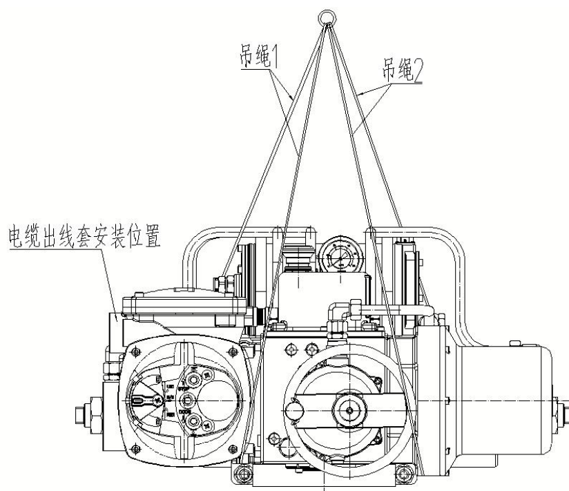
图 4 电液执行机构吊装示意图
