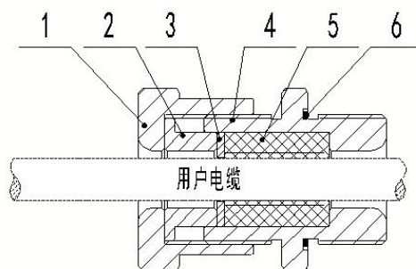
图 5 进线装置
