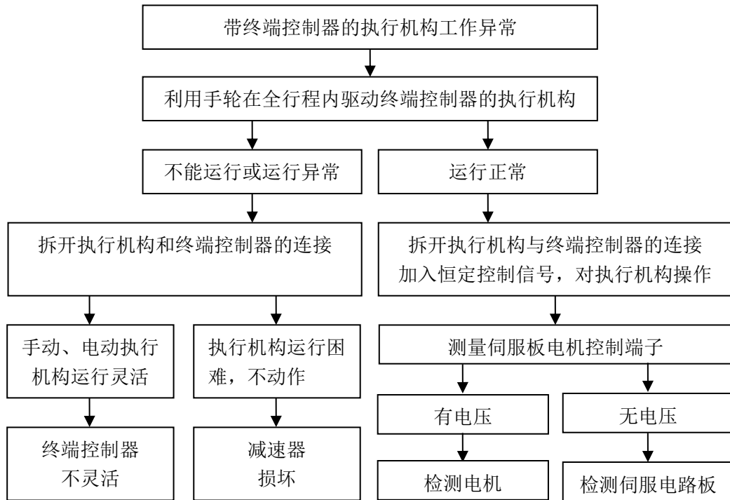
图 14 故障诊断流程
