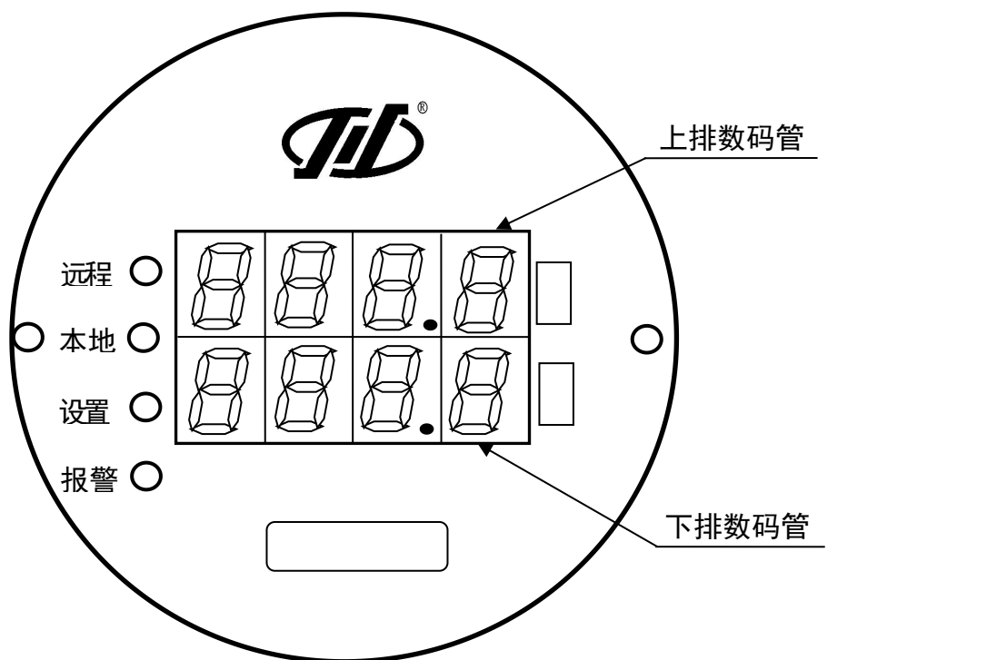
图 12-1 英文显示器（默认）示意图
