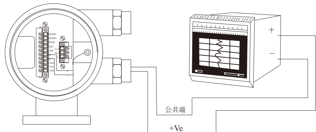
标准型电流输出接线图
