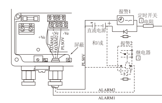
报警接线2
