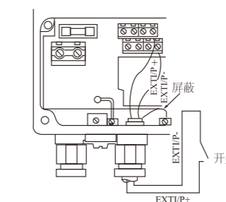
电压信号/逻辑信号
