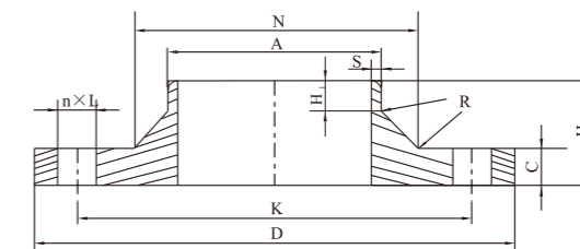
平面(F)对焊钢制管法兰
