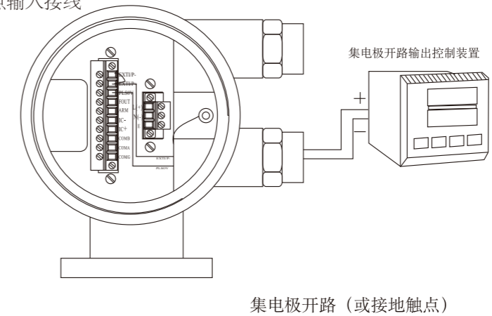
F、触点输入接线
