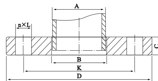
平面 (FF) 板式平焊钢制管法兰
