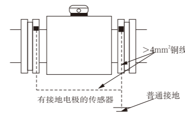
A、金属管道接地
