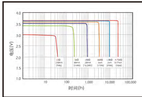
1、在+25℃时的典型放电曲线图（中间值）
