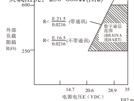
图2 电源电压和外部负载阻抗的关系 电源线的电阻计算公式 R = \rho \frac{L}{S} 电源线线径长短的选择必须符合转换器最低工作电压要求
