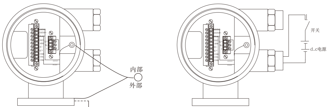
直流供电电源连接图(DC24V)
