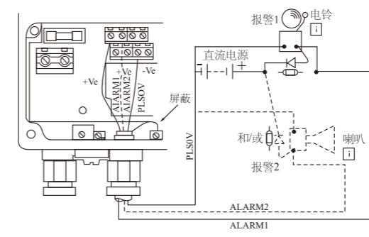
报警接线1
