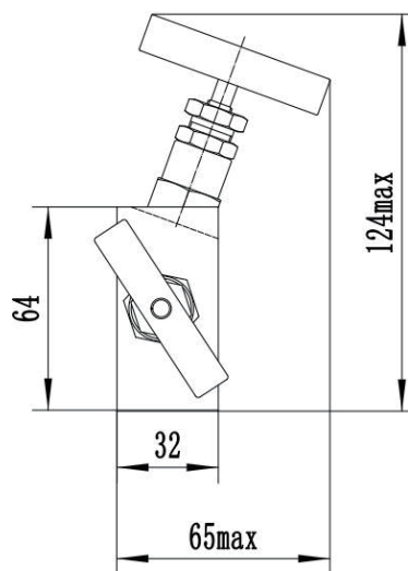
三阀组
