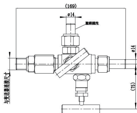
二阀组
