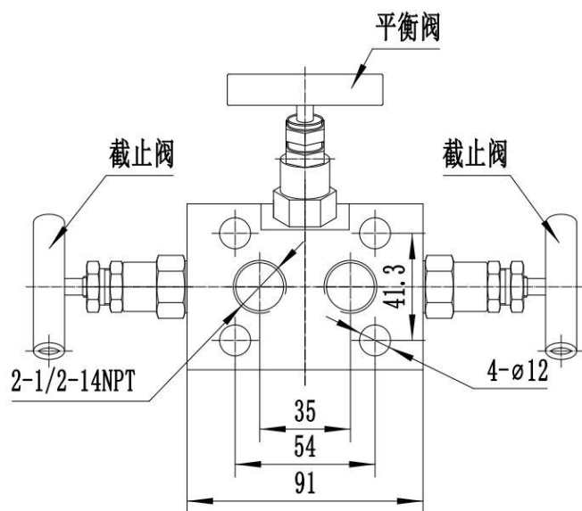
三阀组
