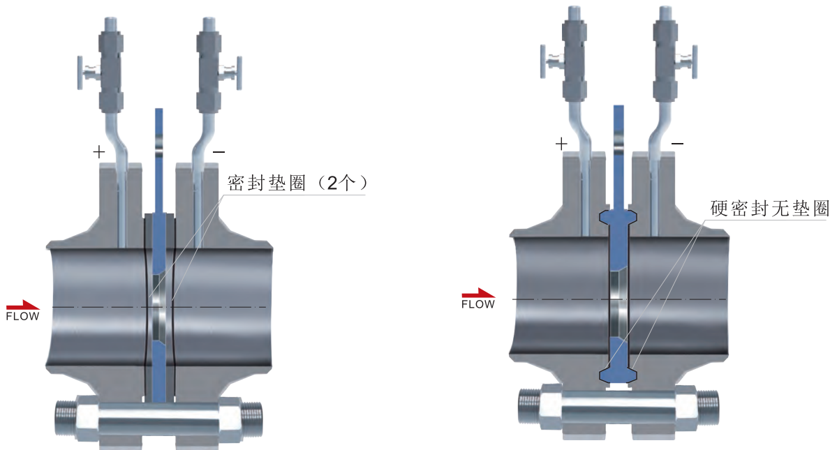
RF平面密封面法兰取压孔板
