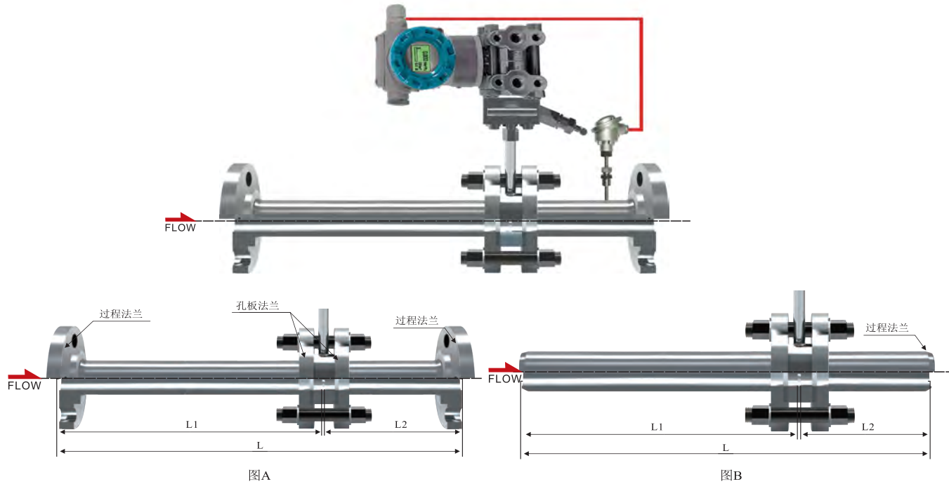
● H型带前后直管段和温压补偿结构示意图
