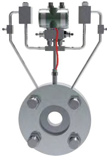
带热电阻补偿及冷凝器 一体化孔板结构
