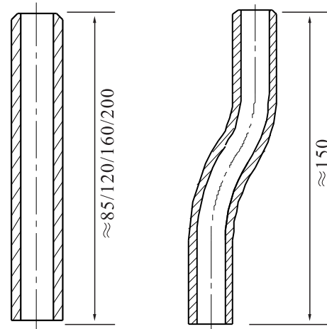
直取压管
