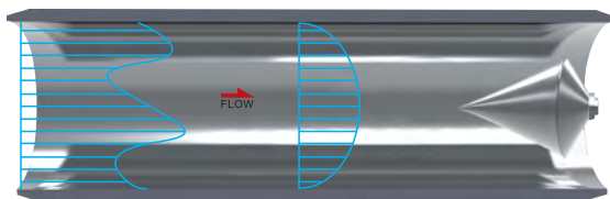
内锥的整流作用
