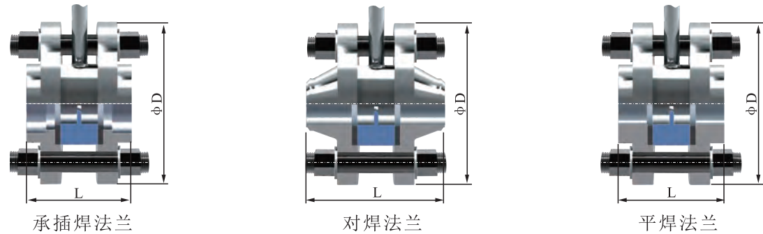
EN 1902-1 (HG20592-97)孔板夹持法兰外形尺寸
