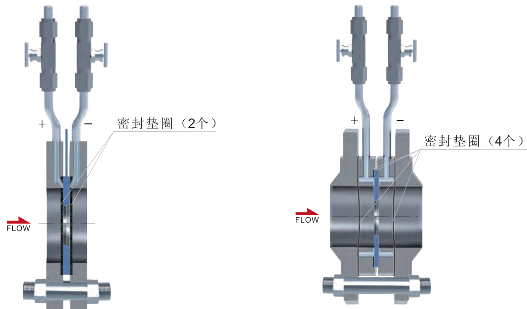
钻孔取压孔板
