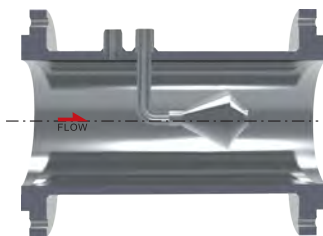
(1) 法兰连接型
