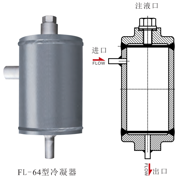
FL-64型冷凝器
