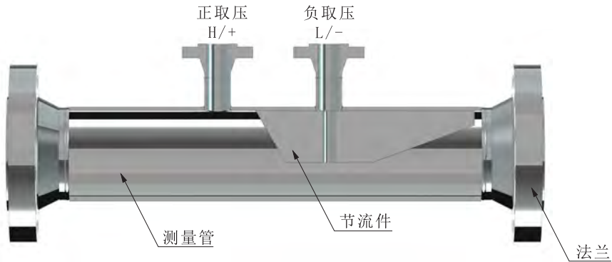
矩形流量计结构图
