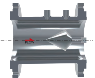
(3) 法兰卡装型
