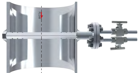
气体安装
