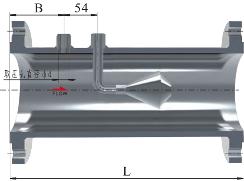
(1) 法兰连接型
