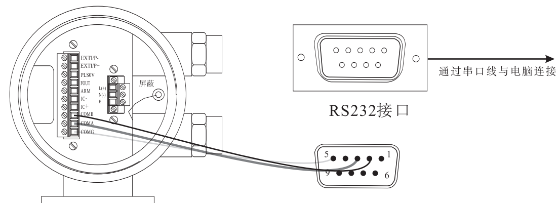
A、RS232接线
