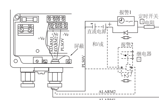
报警接线2
