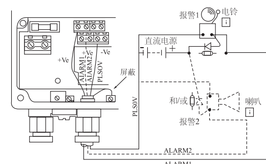
报警接线1
