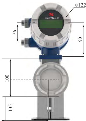
分体型转换器
