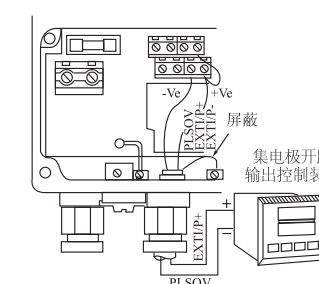
集电极开路（接地触点）
