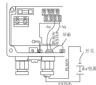
无电压触点
