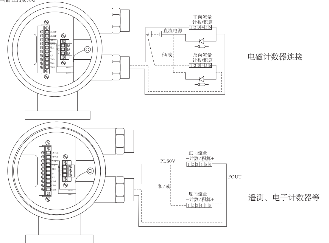
E、报警输出接线
