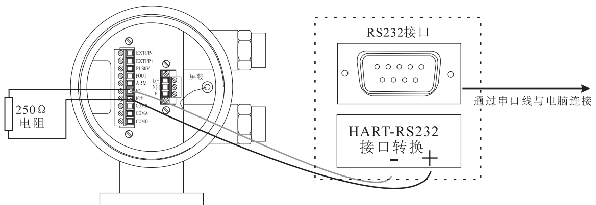
C、HART接线
