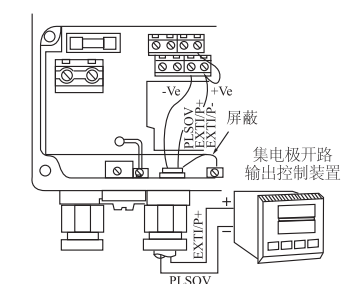
集电极开路（接地触点）
