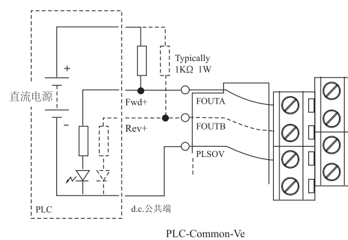
PLC可编程控制器接口示意图（-Ve为公共端）
