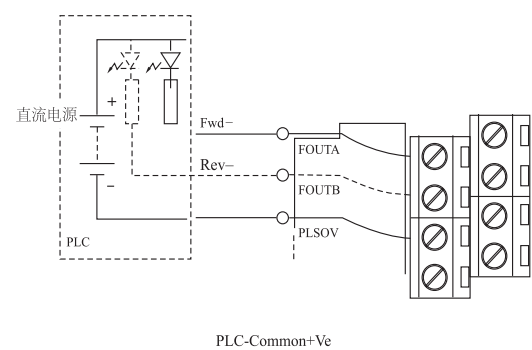
PLC可编程控制器接口示意图（+Ve为公共端）
