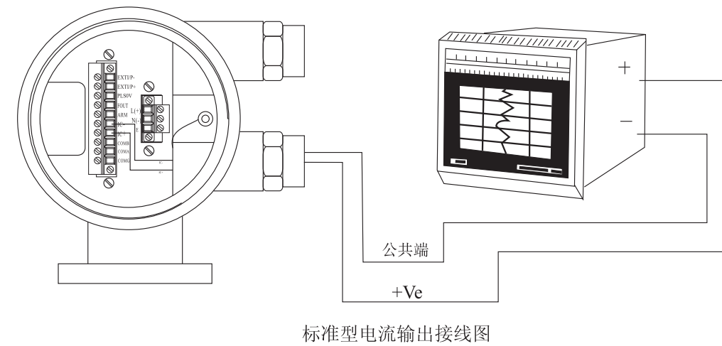
H、电流输出接线
