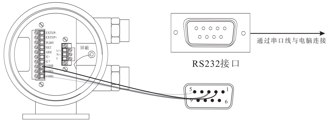
A、RS232接线
