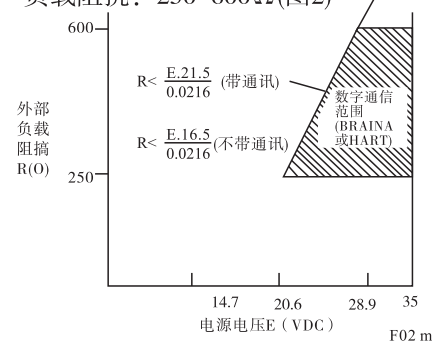
图2 电源电压和外部负载阻抗的关系
