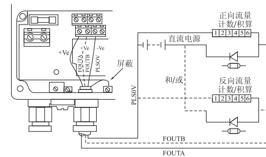
电磁计数器连接
