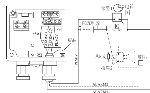
报警接线1
