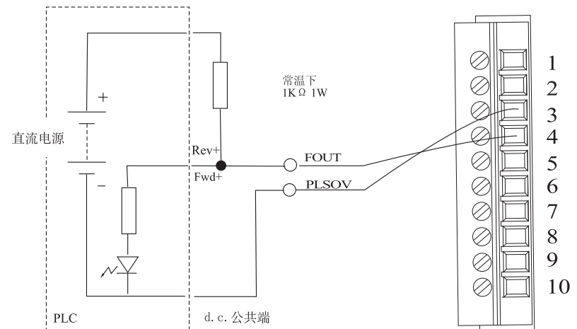
PLC可编程控制器接口示意图 (-Ve为公共端)
