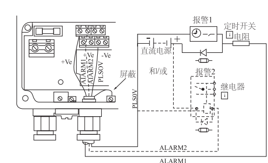
报警接线2
