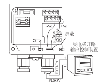
集电极开路（接地触点）
