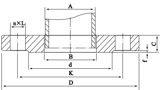
突面 (RF) 板式平焊钢制管法兰
