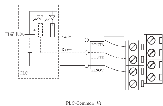
PLC可编程控制器接口示意图（+Ve为公共端）
