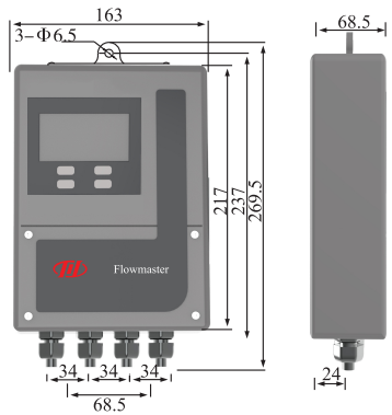
分体式
