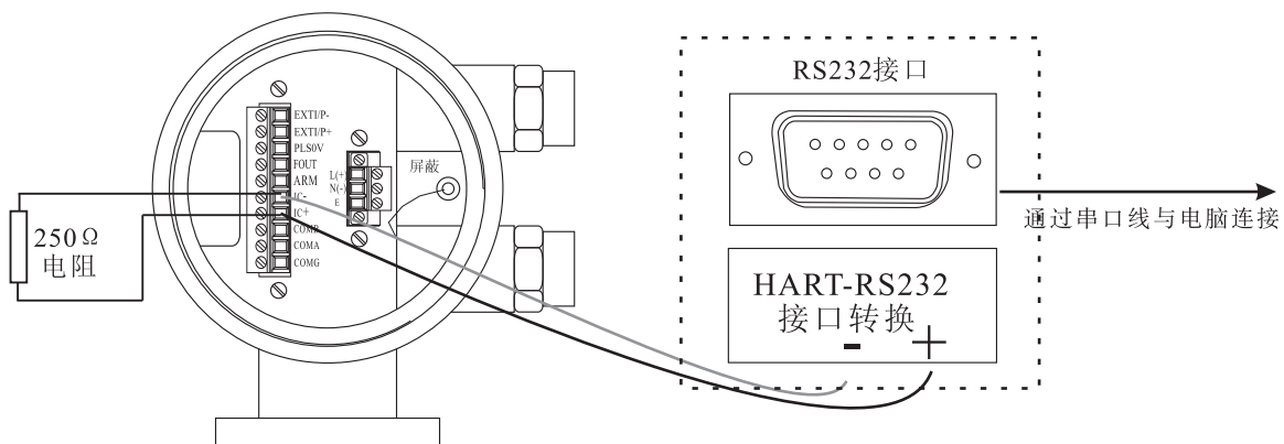
C、HART接线
