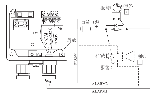
报警接线1
