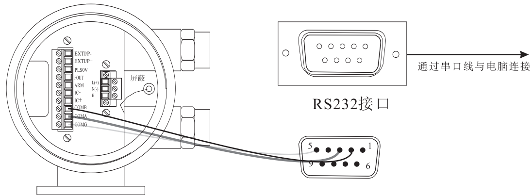
A、RS232接线
