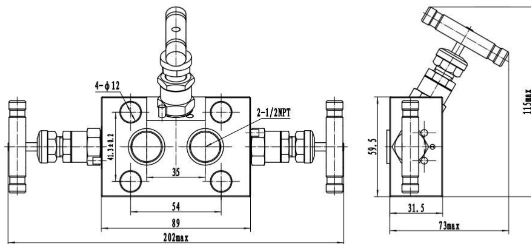
SICV 三阀组
