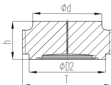
IDF-ISO2853外螺纹接头型
