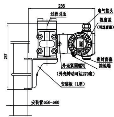
垂直配管安装方式 (安装管垂直)
