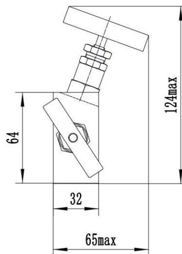
三阀组
