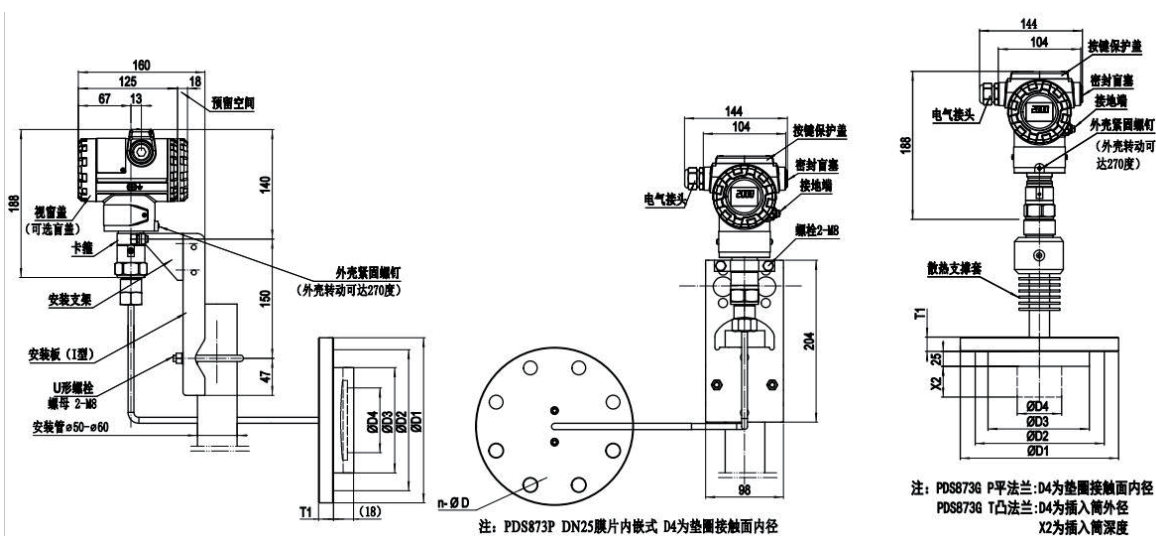
水平配管安装方式 (安装管垂直)
