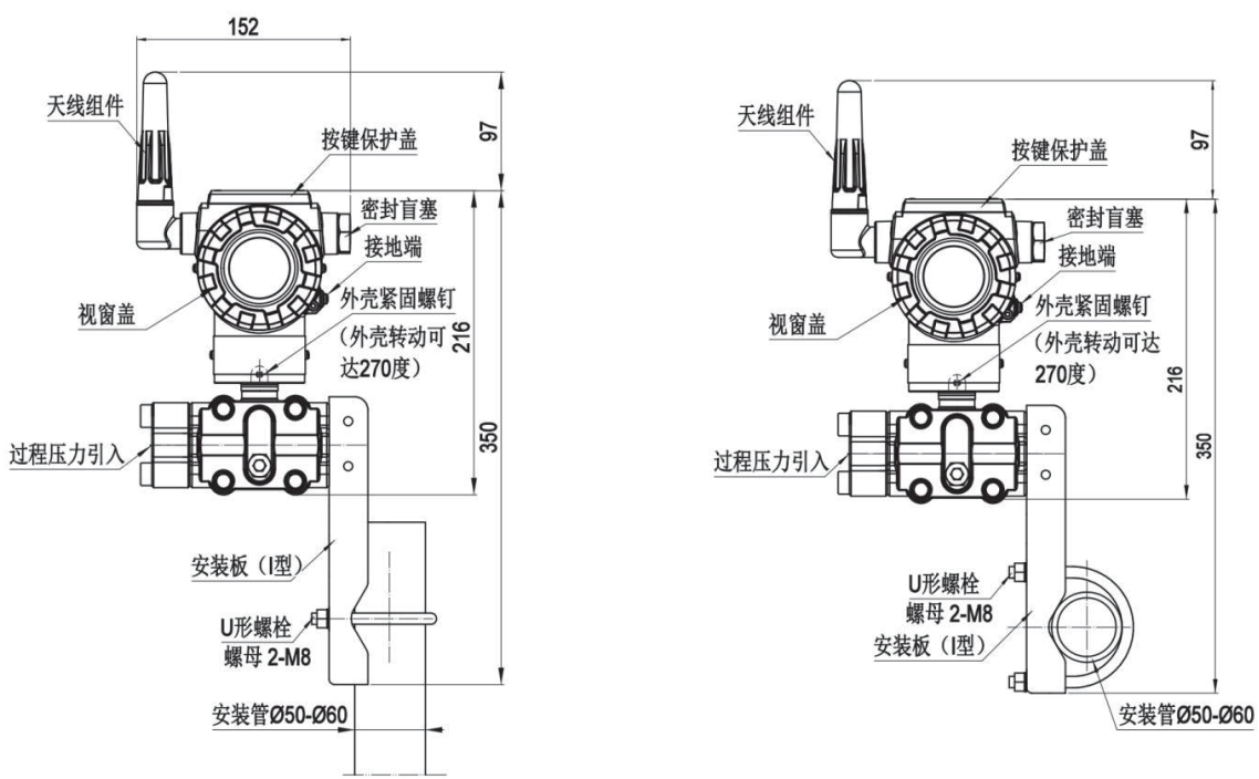
a) 水平配管安装方式 (安装管垂直)
