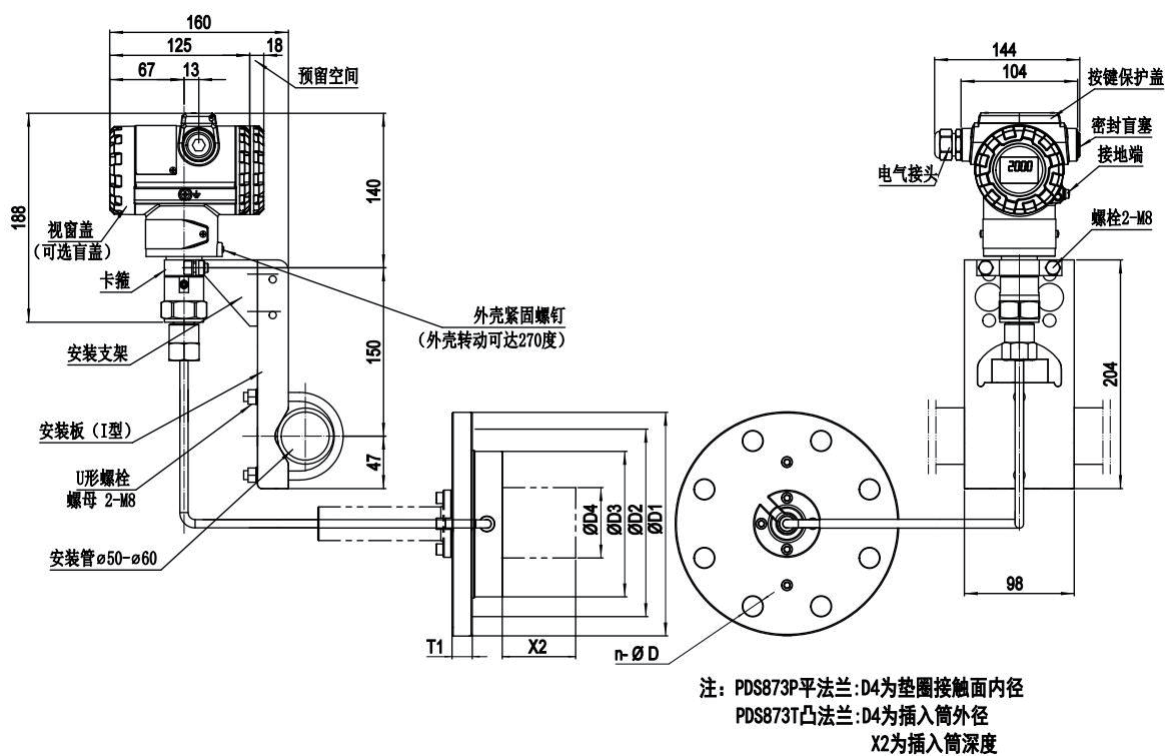
水平配管安装方式 ( 安装管水平)
