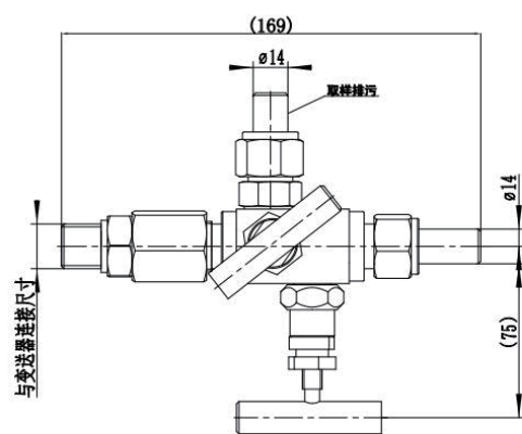
二阀组
