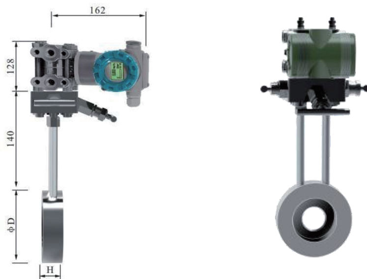
标准孔板结构
