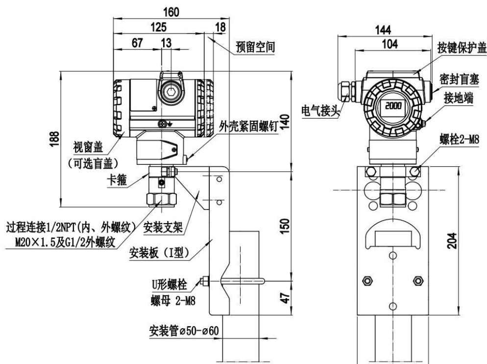
水平配管安装方式 (安装管垂直)
