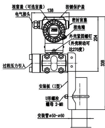
水平配管安装方式 (安装管垂直)
