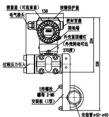
水平配管安装方式 (安装管水平)
