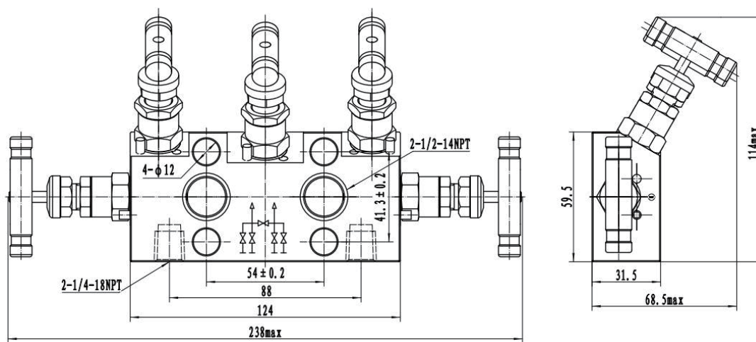
SICV 五阀组
