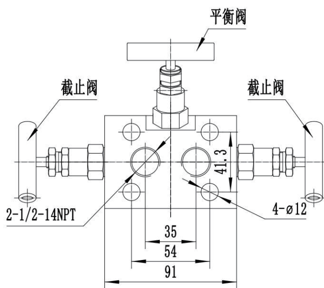
三阀组
