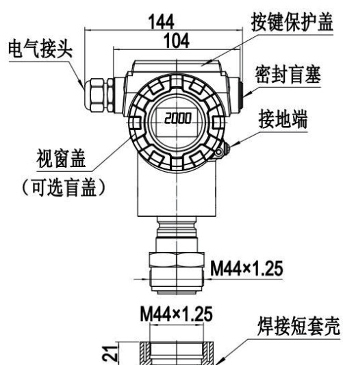
PDS813 M44×1.25 平齐安装
