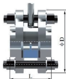
平焊法兰
