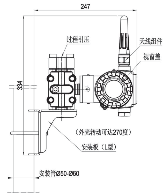
b) 垂直配管安装方式
