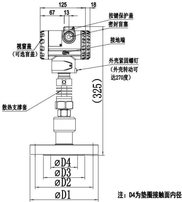
PDS879 超高温远传压力变送器（直连式）
