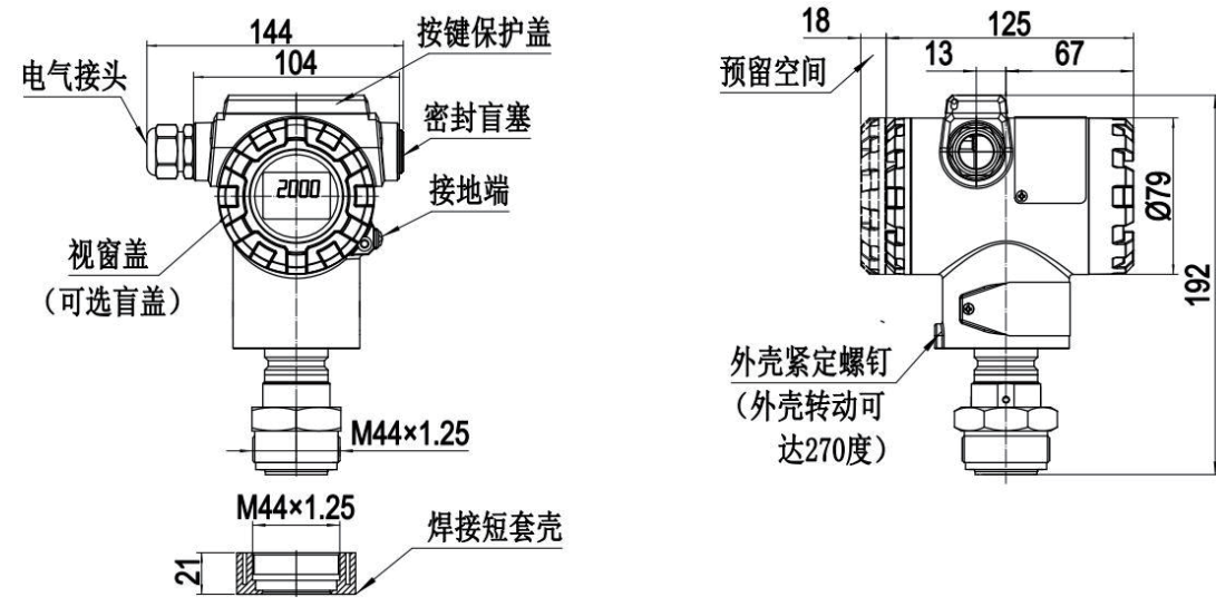
PDS813 M44x1.25 平齐安装
