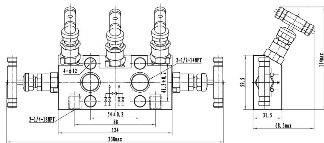
SICV 三阀组
