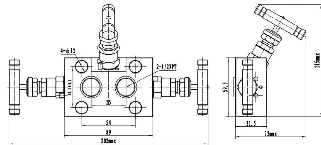
SICV 五阀组
