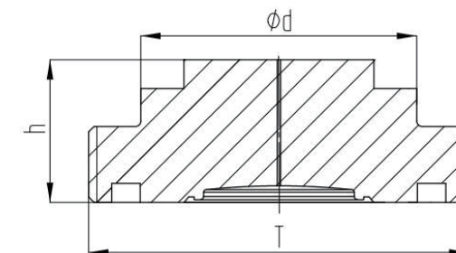
SMS1145外螺纹接头型
