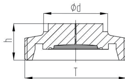
DIN11851外螺纹接头型
