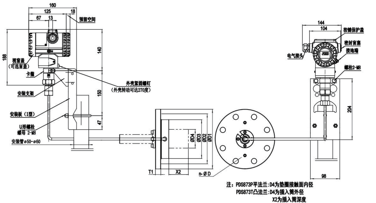
水平配管安装方式（安装管垂直）
