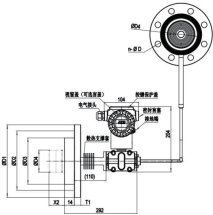
H (正) 側高温直連式
