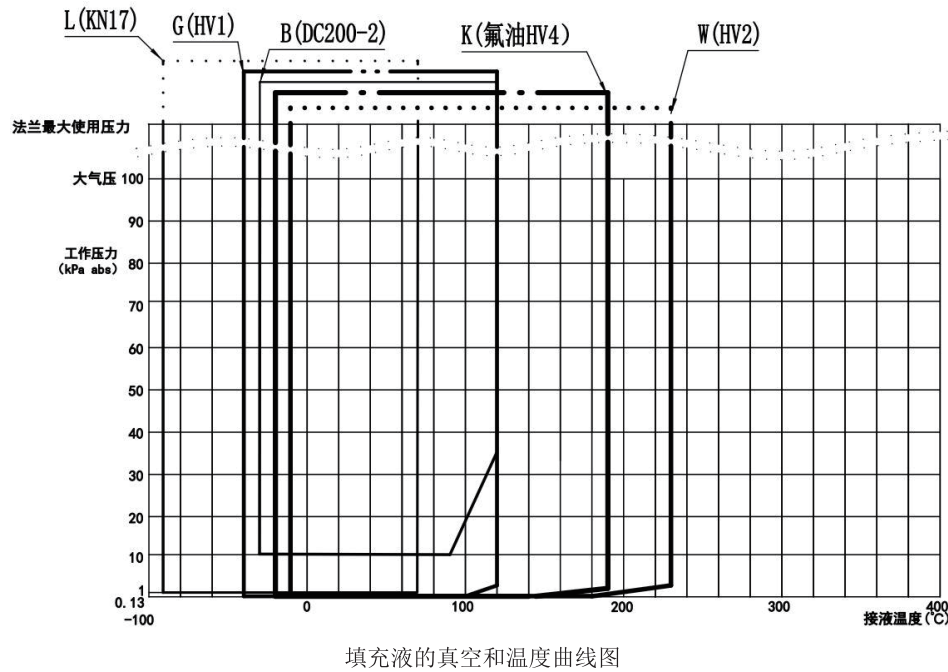
填充液的真空和温度曲线图
