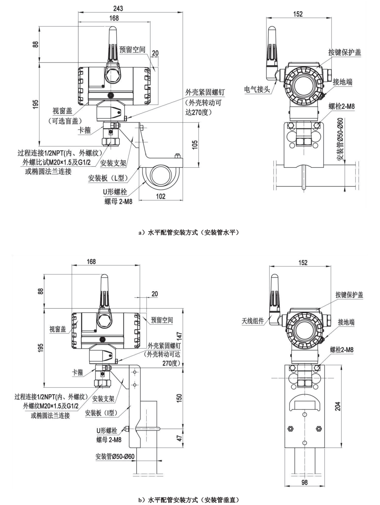
◆PDS800 无线系列压力变送器外形及安装尺寸
