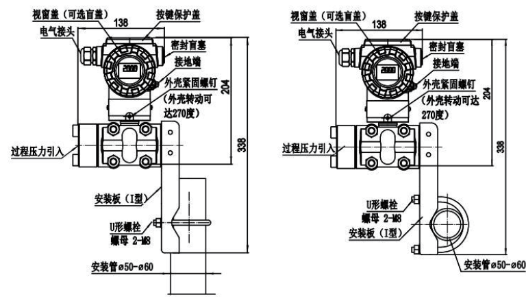
水平配管安装方式 (安装管垂直)
